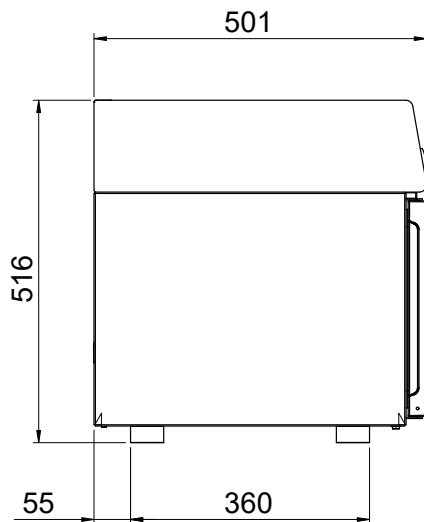
Boven aanzicht
